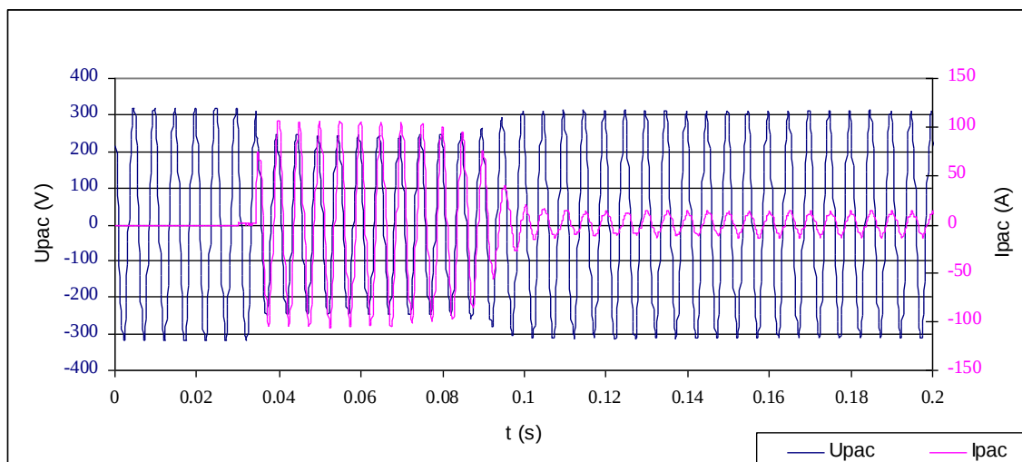
Creux de tension au démarrage d'une pompe à chaleur monophasé
