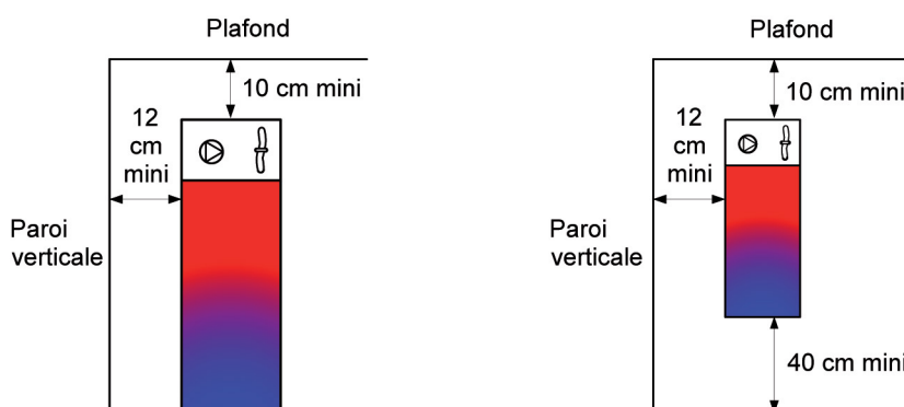
▲ Figure 6 : Espaces libres minimaux à réserver autour du chauffe-eau thermodynamique pour une installation au sol et murale (selon le NF DTU 60.1 P1-1-3)
