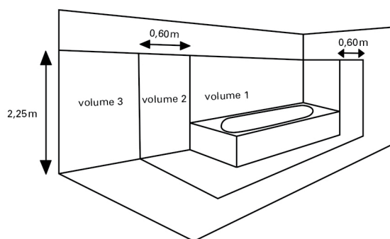
▲ Figure 5 : Volumes de sécurité définis dans la norme NF C 15-100
