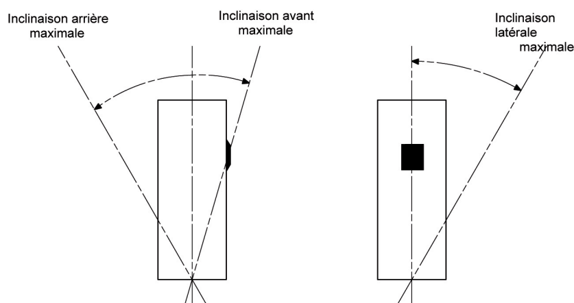
▲ Figure 4 : Tolérance d'inclinaison des chauffe-eau thermodynamiques sur les différentes orientations
