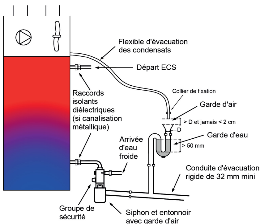
▲ Figure 9 : Schéma de principe du raccordement hydraulique d'un chauffe-eau thermodynamique
