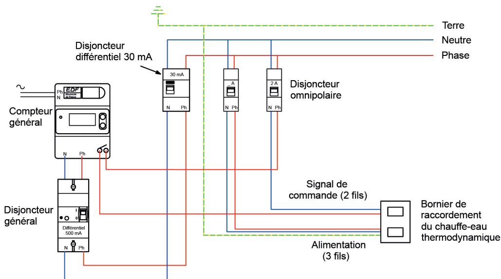
▲ Figure 7 : Raccordement électrique dans le cas d'un asservissement temporel par le signal tarifaire du compteur électrique
