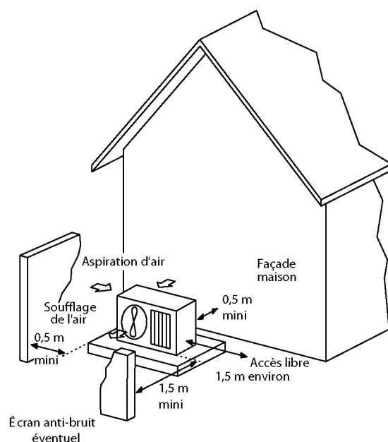
▲ Figure 12 : Exemple d'implantation de l'unité extérieure du chauffe-eau thermodynamique
