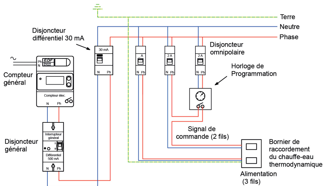
▲ Figure 8 : Exemple de raccordement électrique dans le cas d'un asservissement temporel par une horloge de programmation externe
