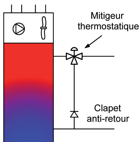
▲ Figure 10 : Mise en place d'un clapet anti-retour si un mitigeur thermostatique est installé juste en sortie de production
