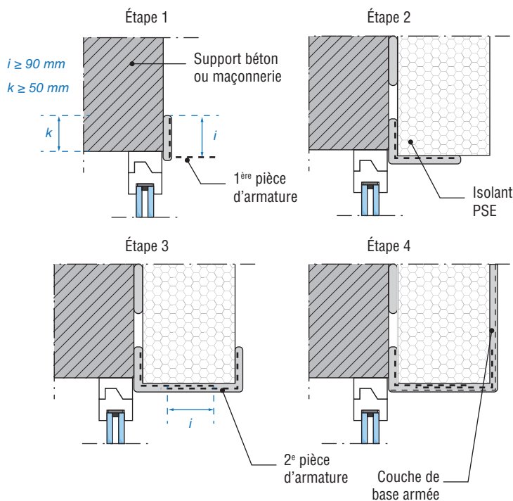
Figure 8 : Solution B – Phasage de la mise en œuvre des paniers renforcés : cas d'une menuiserie en tunnel au nu extérieur du gros œuvre
