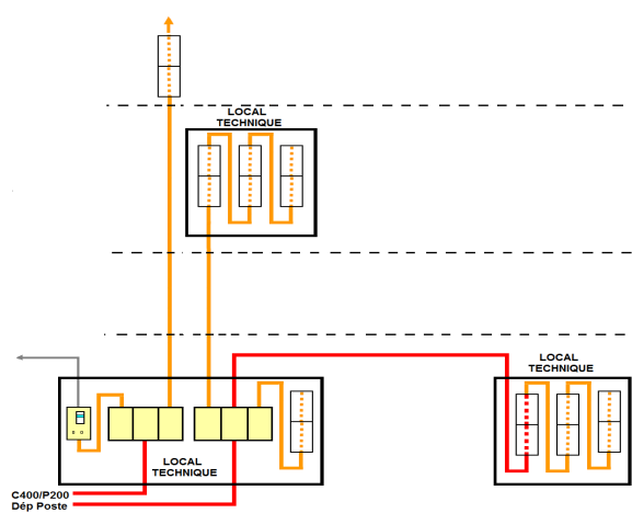
2-8 Locaux techniques et colonne(s)
