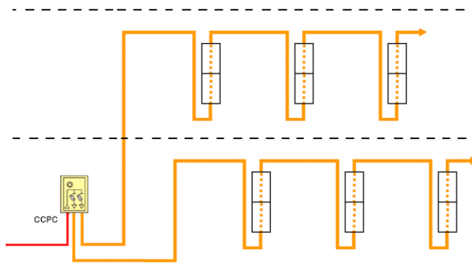
2-2 Double Colonne Horizontale (Distributeurs dans gaine *)
