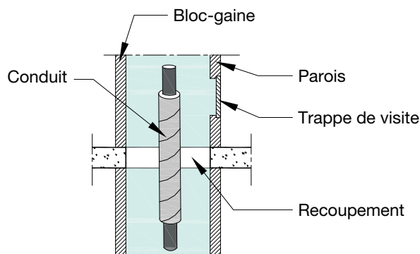
RECOUPEMENT DANS GAINÉ TRAVERSANTE
