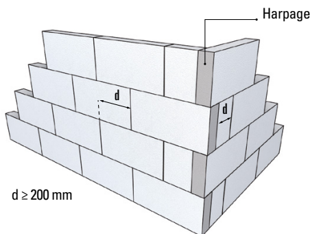
Pose de panneaux isolants à joints décalés et harpage aux angles
